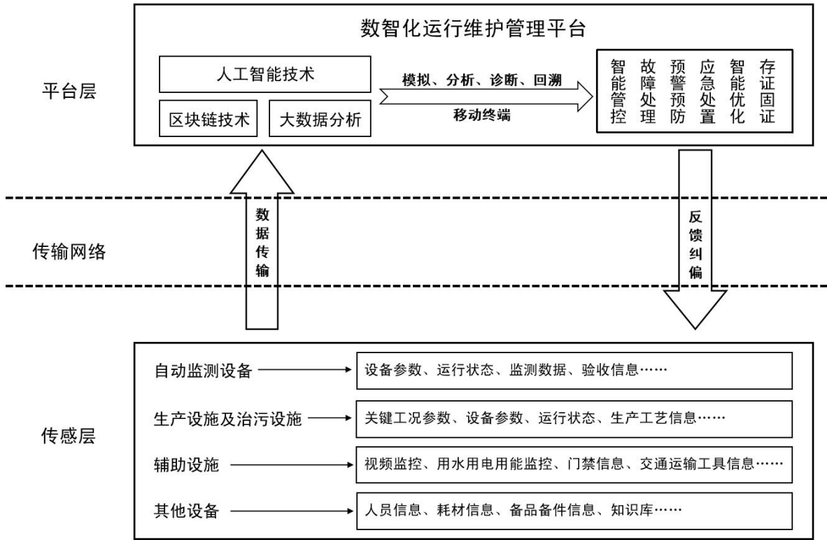
图 1 数智化运行维护系统架构图
